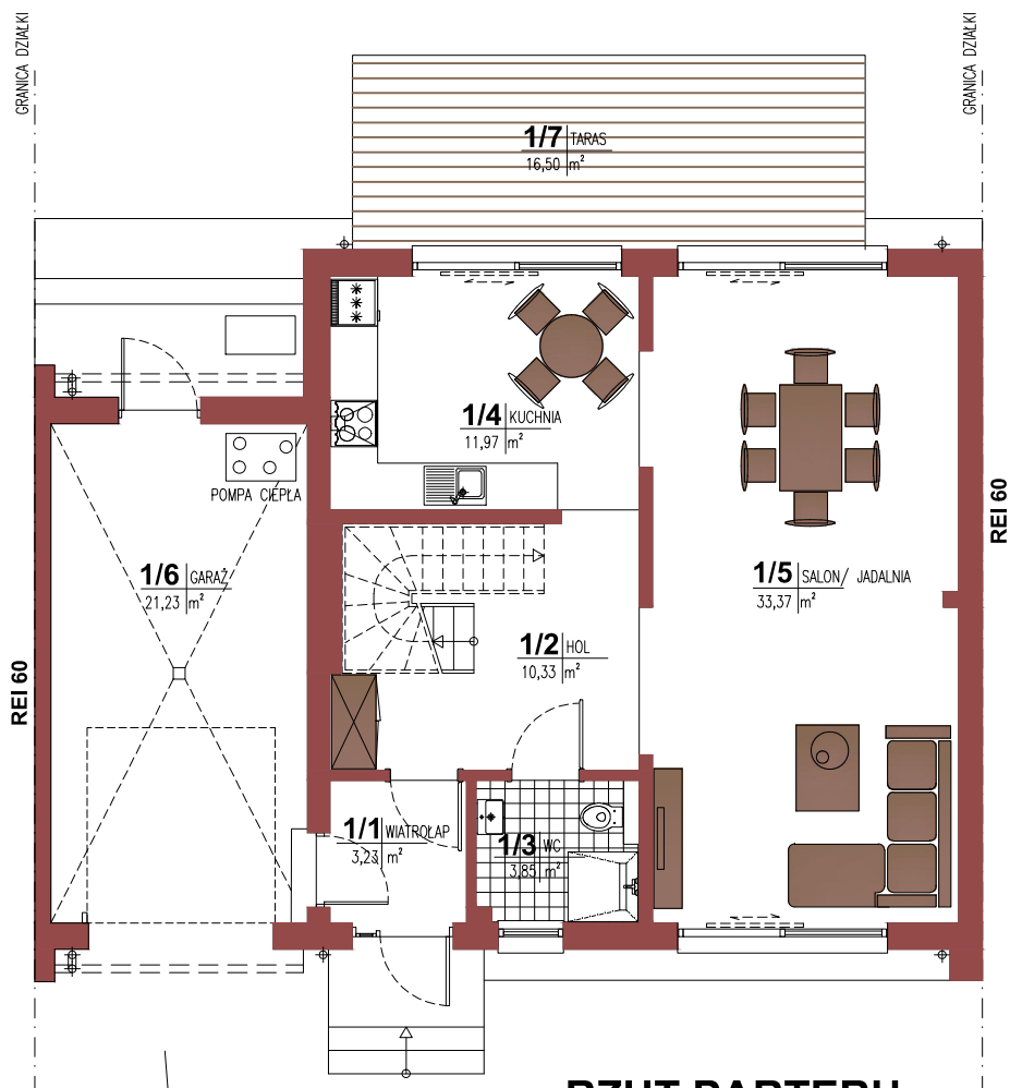
RZUT PARTERU
