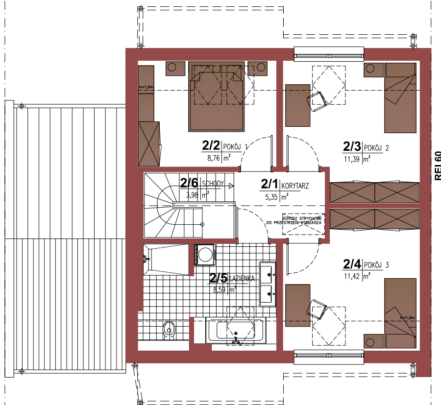
RZUT PODDASZA
