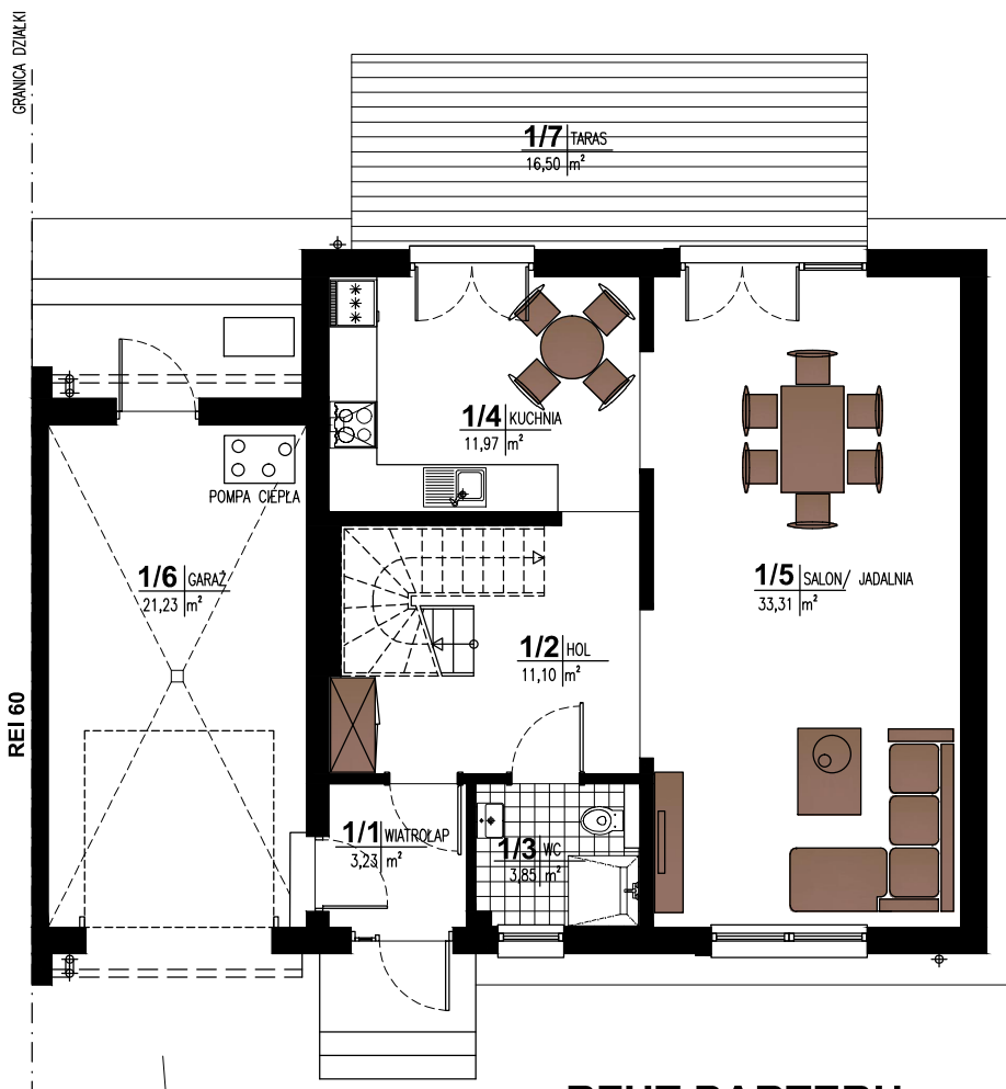
RZUT PARTERU
